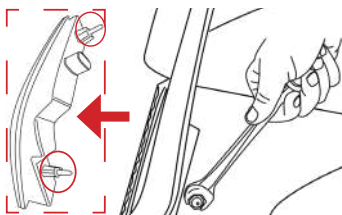
VISTA TRASEIRA DLR
